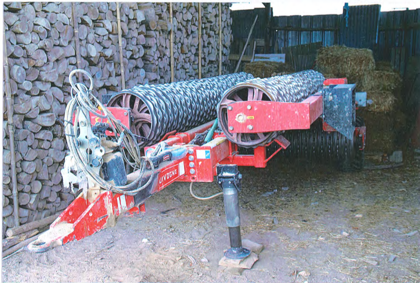
Rouleau autoporteur
